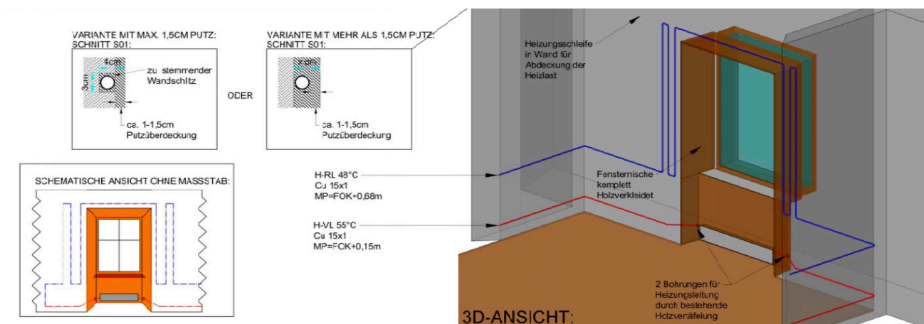
Bauteilheizung
